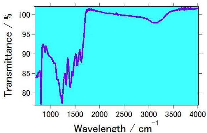
グラファイト状窒化炭素(g-C 3 N 4 )の FT-IR
