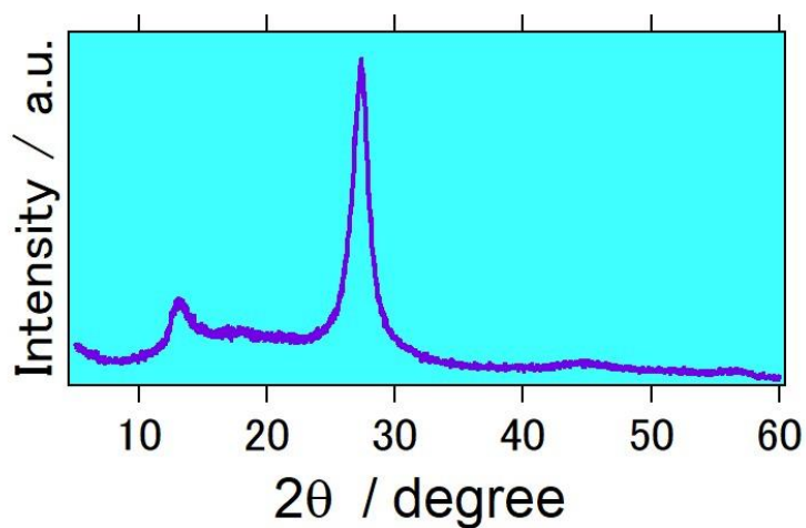
グラファイト状窒化炭素(g-C 3 N 4 )の XRD
