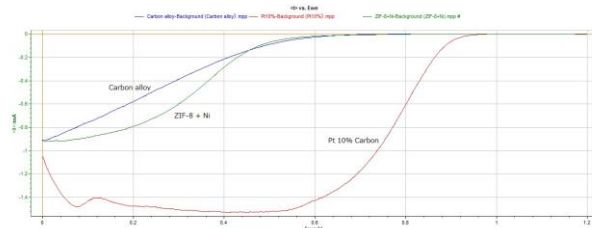
回転電極を用いて測定した触媒電極活性(上からカーボンアロイ系触媒、MOF系触媒、白金担持触媒)
